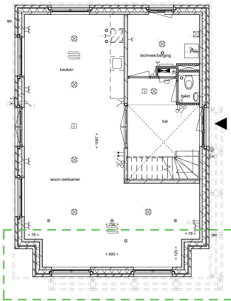
begane grond
