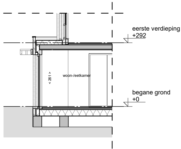
code 10130: uitbouw achtergevel 120cm
